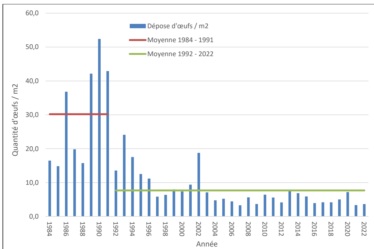
Fig. 12 : Evolution de la dépose d'œufs de 1984 à 2022 (nombre/m²)
